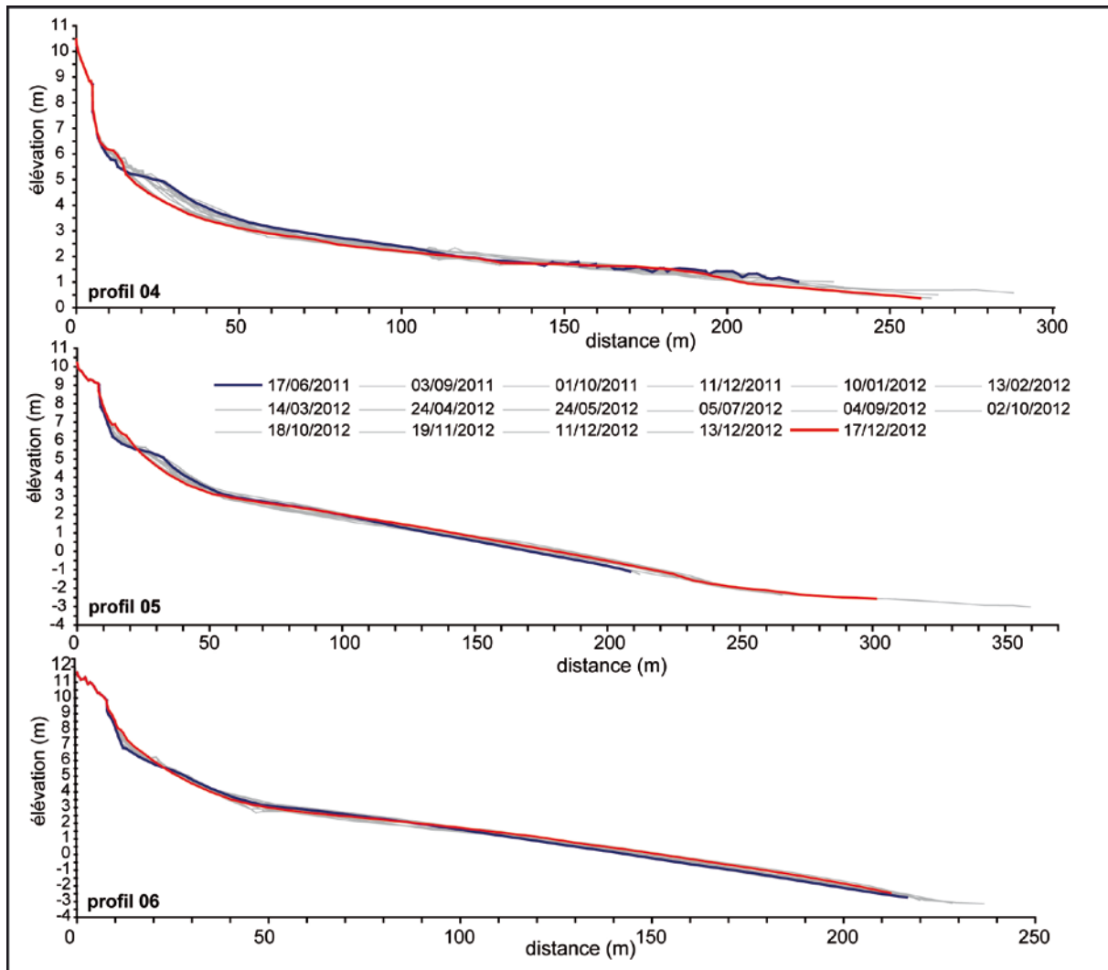
Figure 3 (suite) – Enveloppes de profils de plage / dune pour les radiales 4, 4 et 6, entre les mois de juin 2011 et de décembre 2012
